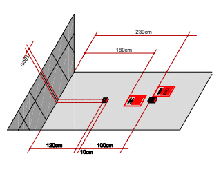
SINALIZAÇÃO DO ALARME DE INCÊNDIO
